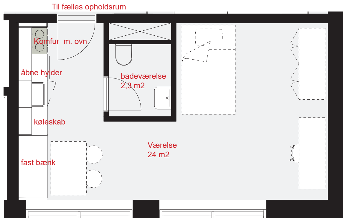
BOLIGTYPE D 1:50
